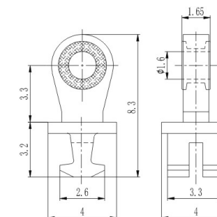
加胶铰链 Safely hinge
