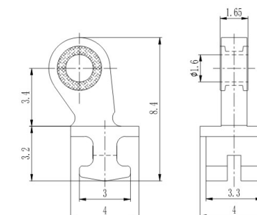
加胶铰链 Safely hinge
